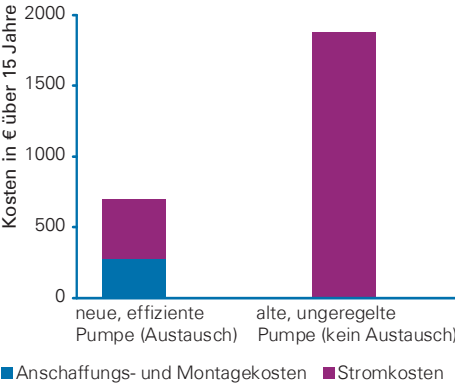
Kostenvergleich Heizungspumpe neu und alt
