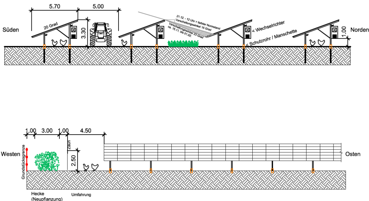
Abbildung 8 - Systemschema einer möglichen Konstruktion
